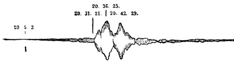
16: Fig. 16. — I Shide upptaget seismogram.
