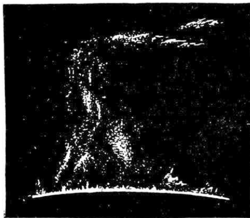
21: Fig. 21. — Rökpelarförmad lugn protuberans.
