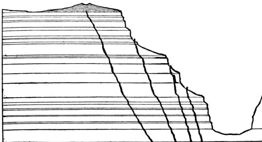
8: Fig. 8. — Lavafyllda sprickor med en vulkanisk askkägla på Torowheap-canon, Coloradoplåtan. Skematisk bild.
