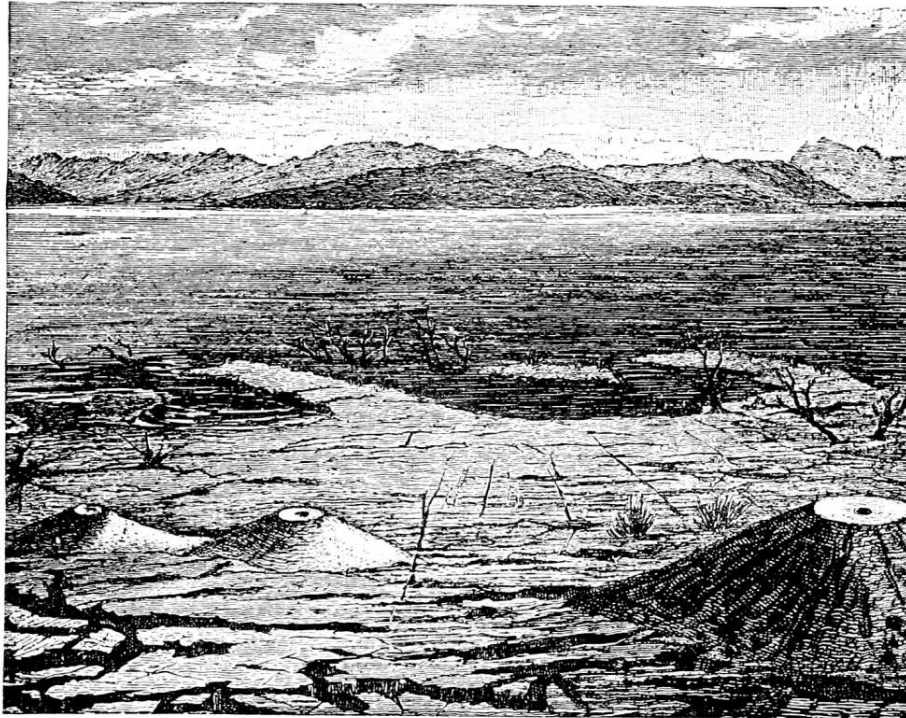
12: Fig. 12. — Sandkratrar och sprickor bildade vid jordskalfvet vid Korint 1861. I vattnet grenar från översvämmade träd.
