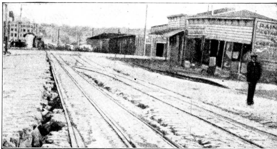
11: Fig. 11. — Sprickor i Valentia Street, S. Francisco efter jordbäfningsen år 1906.
