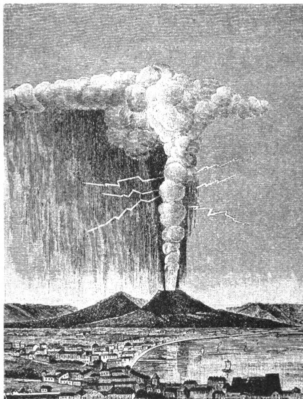
3: Fig. 3. — Vesuvii utbrott år 1822 efter en samtida handteckning.
