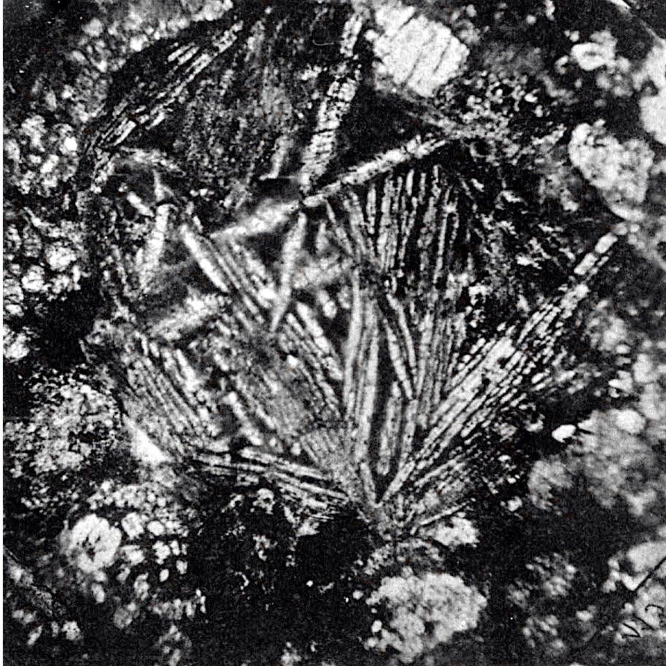
106: Tafel 26: Figur 6 — auf Knyabinya D. 2,20 mm. (die dunkle Linie in 5 und 6 ist der Nahrungsanal)
