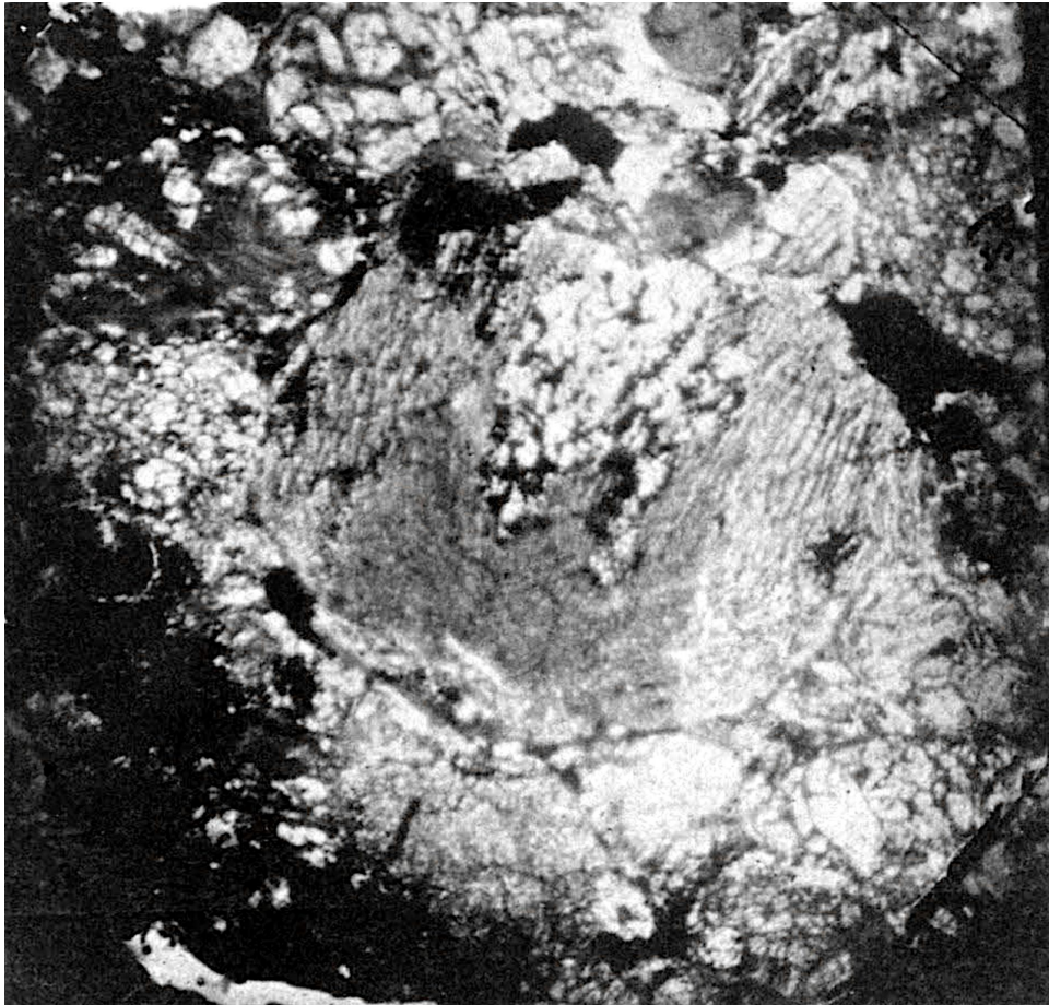
18: Tafel 4: Figur 5 — auf Rnyahinya D. 1,60 mm.
