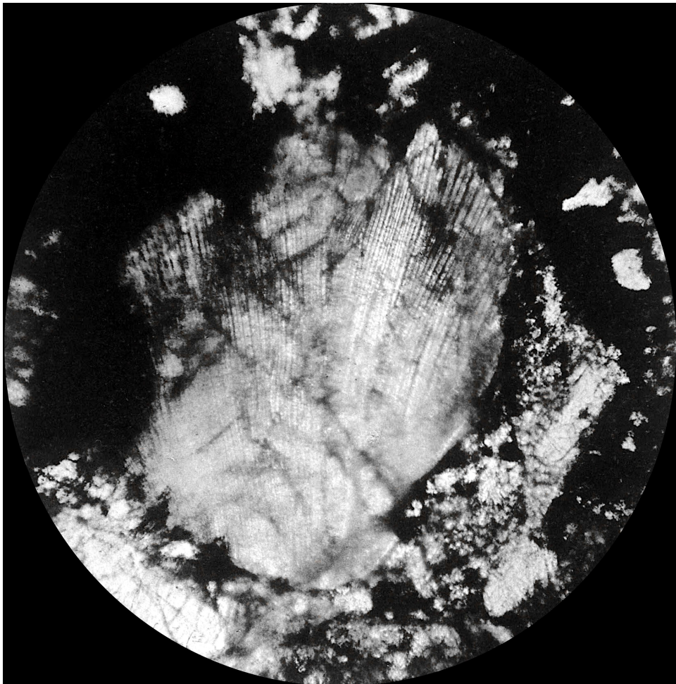
38: Tafel 8: Figur 1 — (Favosites) auf Knyahinya (vergl. Tafel 1: Figur 4)
