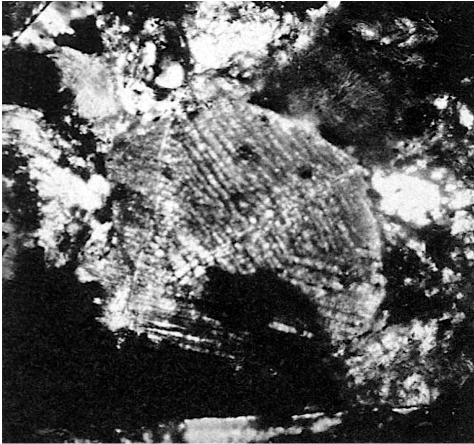
133: Tafel 3I: Figur 3 — auf Knyahinya D. 1,20 mm. (Drei übereinstimmende Formen auf 3 Dünnschliffen, in 1 und 2 beidemale der horizontale Aufschnitt)
