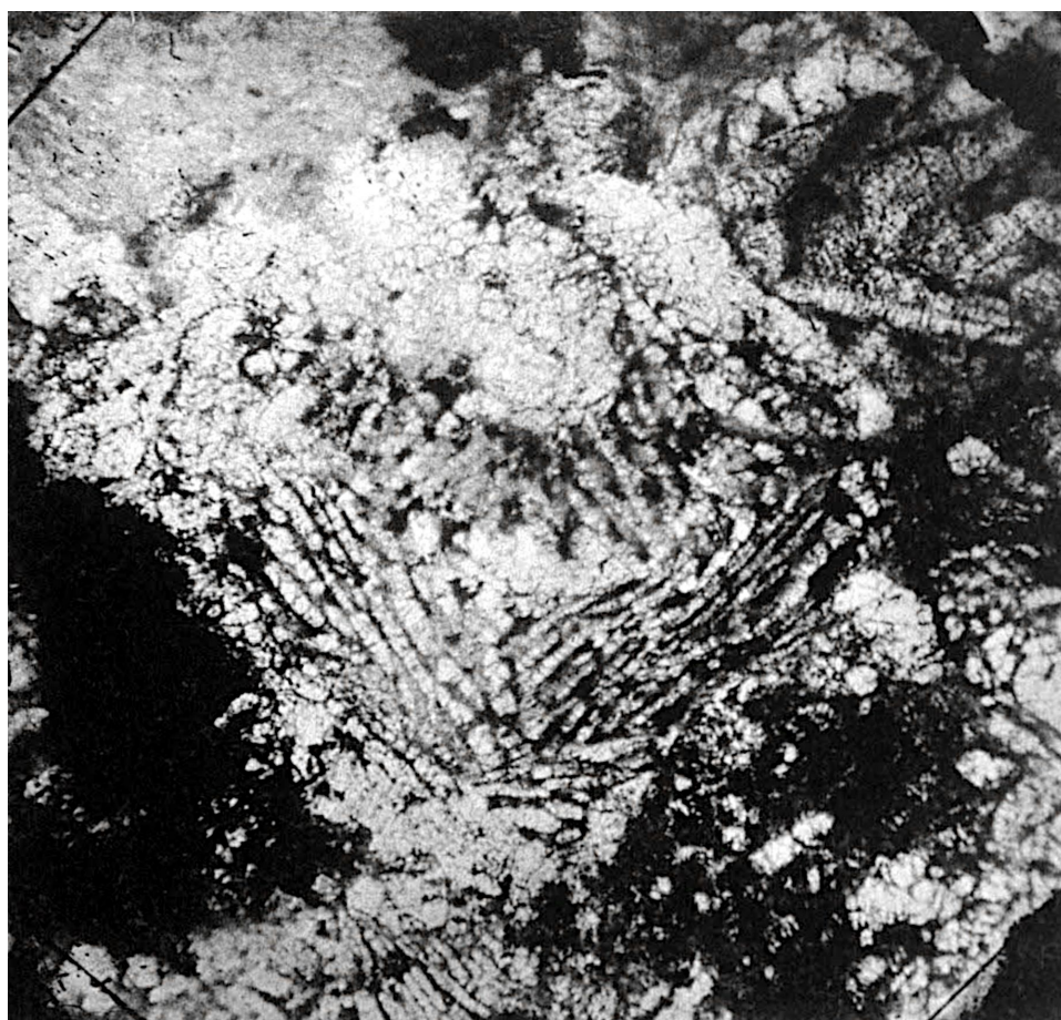
ИІ8: Tafel 28: Figur 6 — auf Knyahinya D. 1,40 mm.
