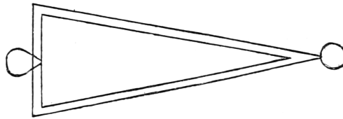
24 - Κέρτακis. — Réduction aux 2/3.
