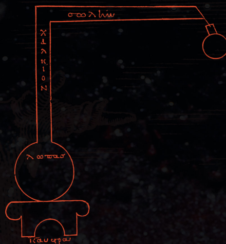
16 – Appareil distillatoire. Réduction aux 2/3.
