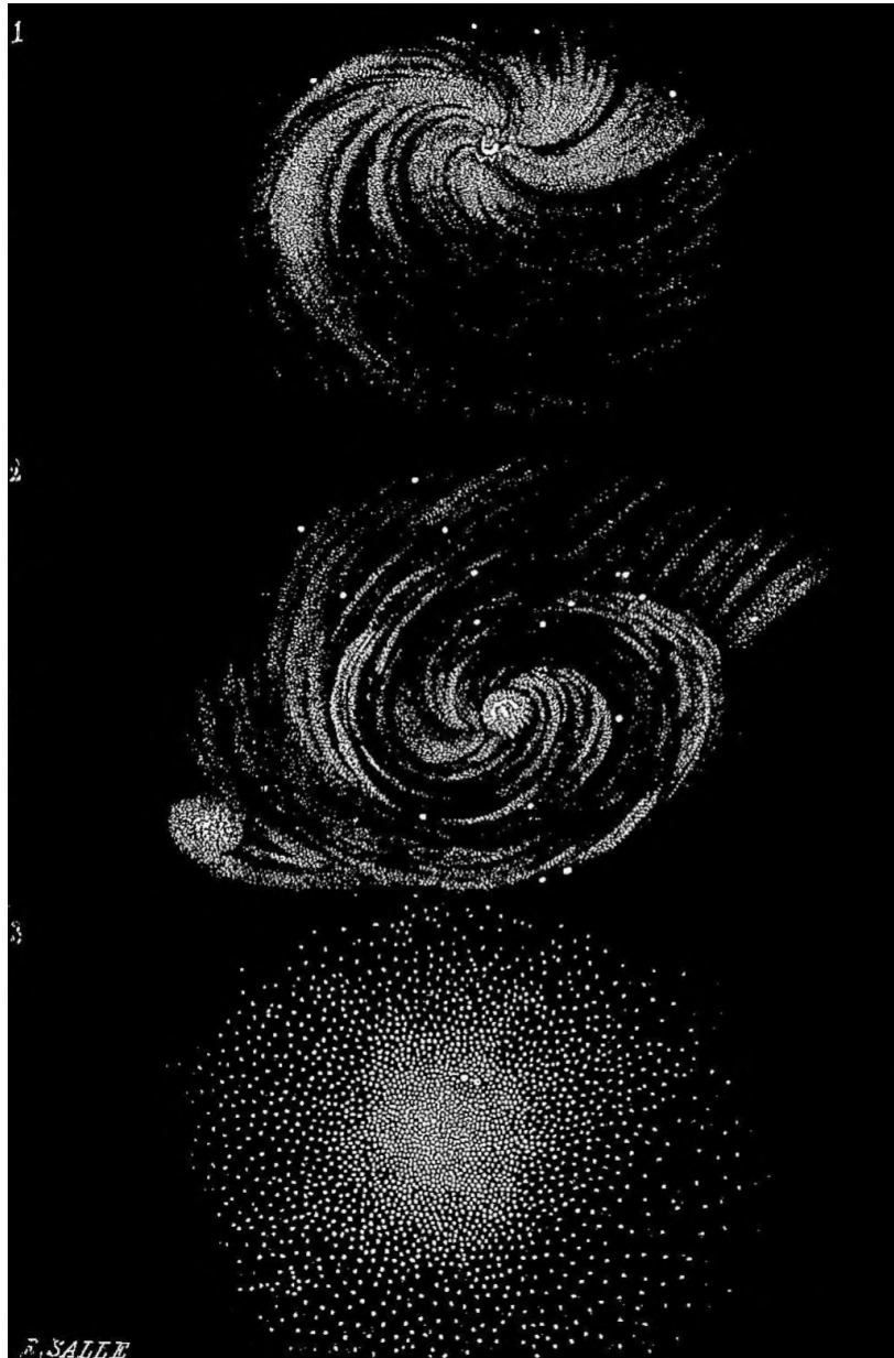
4 - Nébuleuses. — 1. Nébuleuse de la Vierge. — 2. Nébuleuse des Chiens de chasse. — 3. Amas du Coucan.
